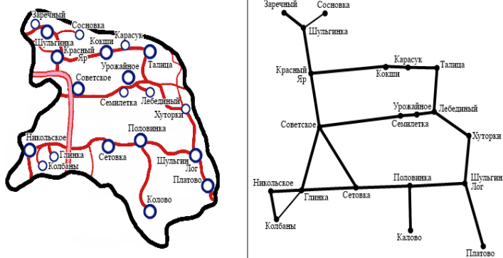
Рисунок 3 – Карта и подграф сети автомобильных дорог Советского района
